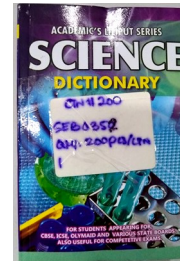
SEB0352 SCIENCE
