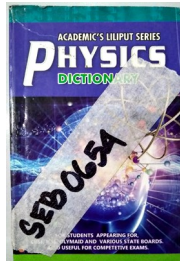
SEB0654 PHYSICS
